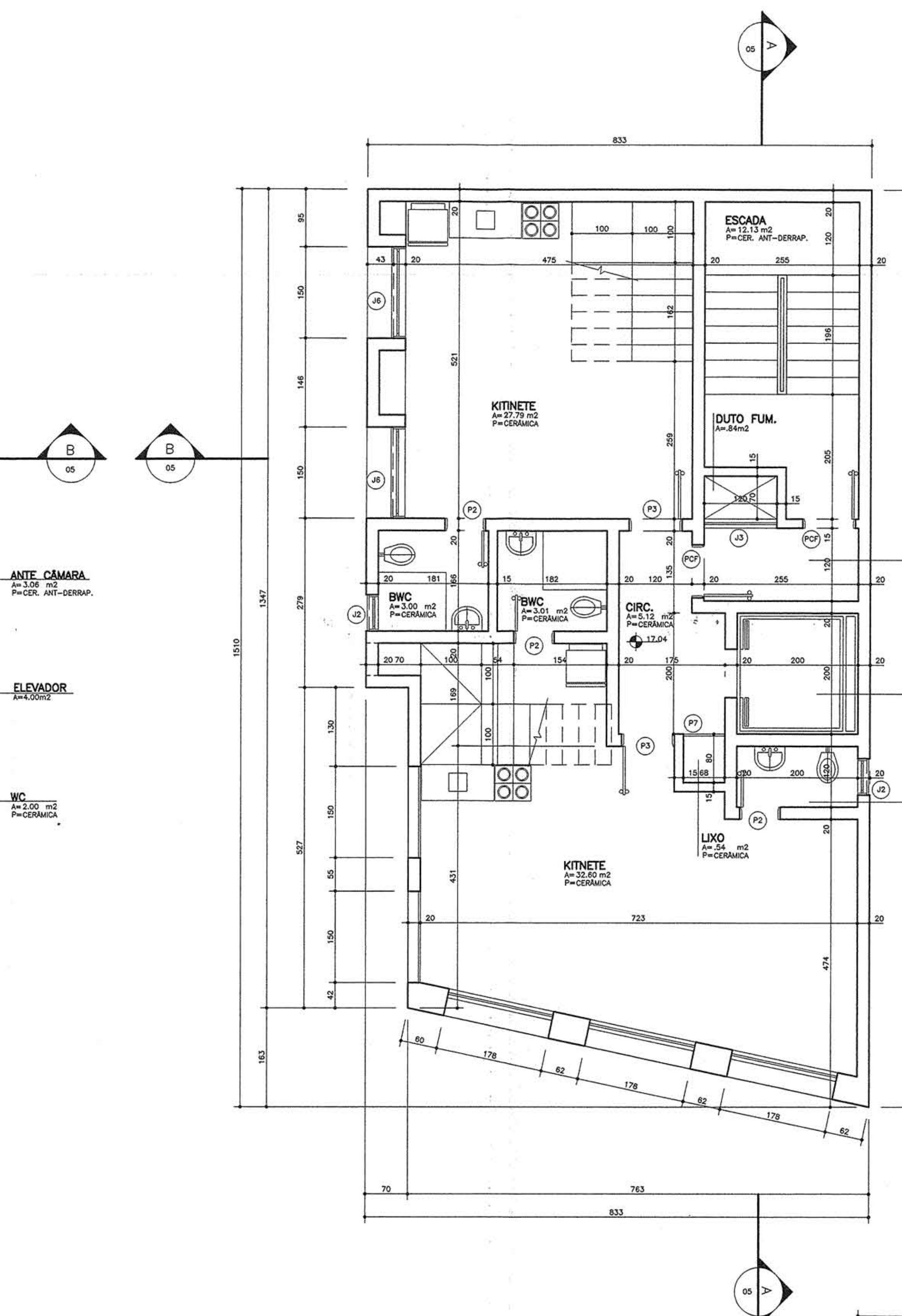
PLANTA BAIXA 5ª PAVTO ESC. 1/50
