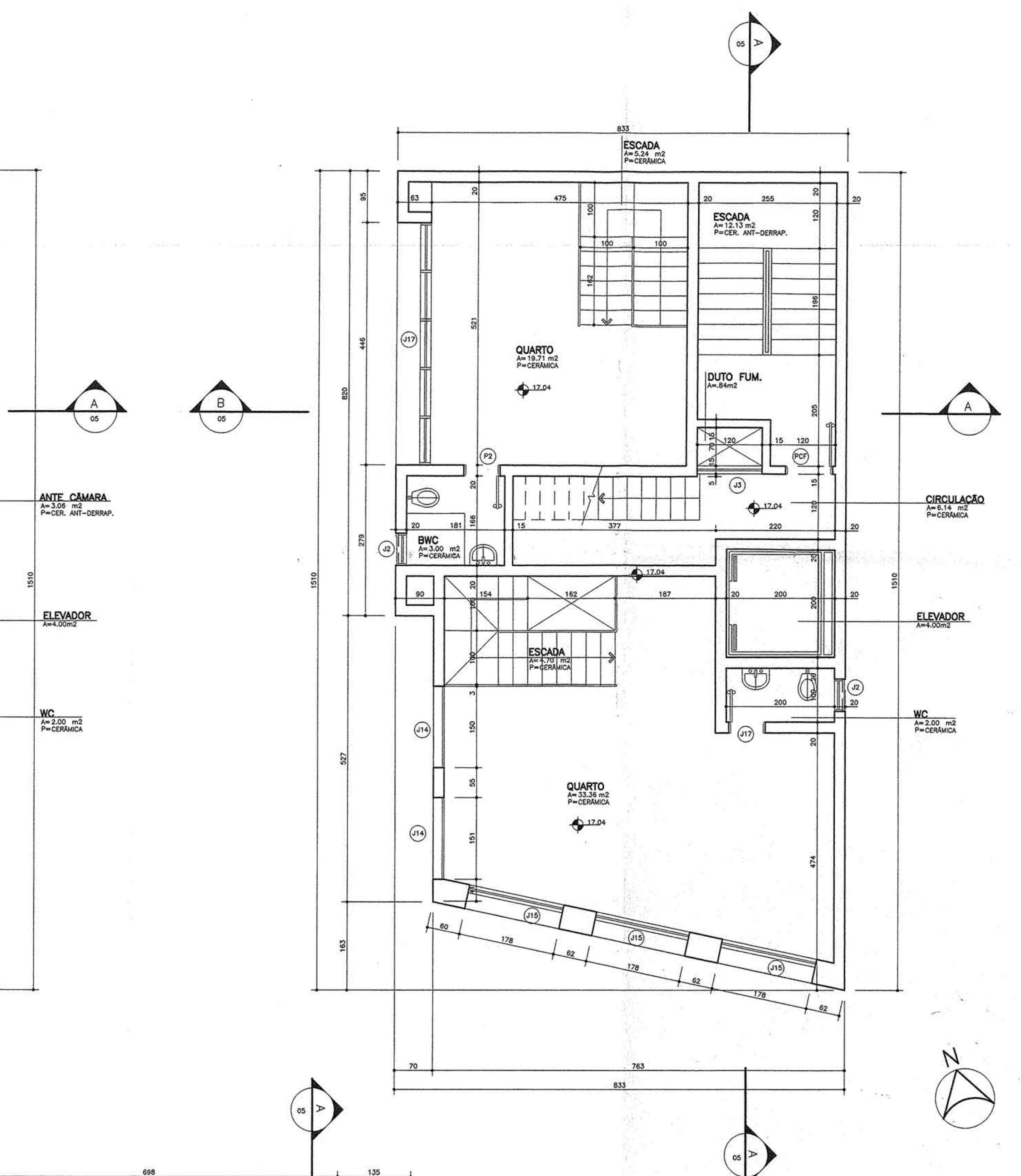
PLANTA BAIXA 6ª PAVTO (DUPLEX) ESC. 1/50
