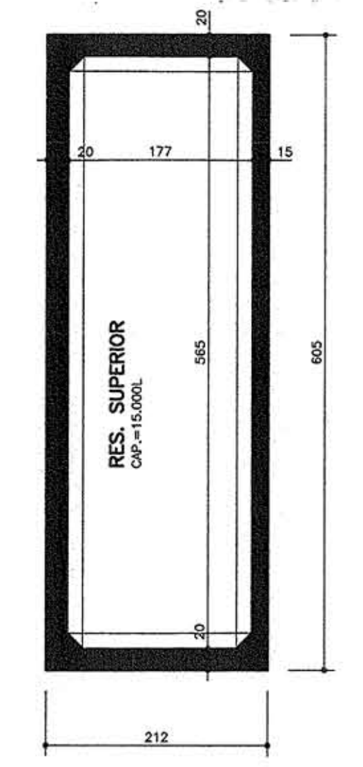
RES. SUPERIOR ESC. 1/50
